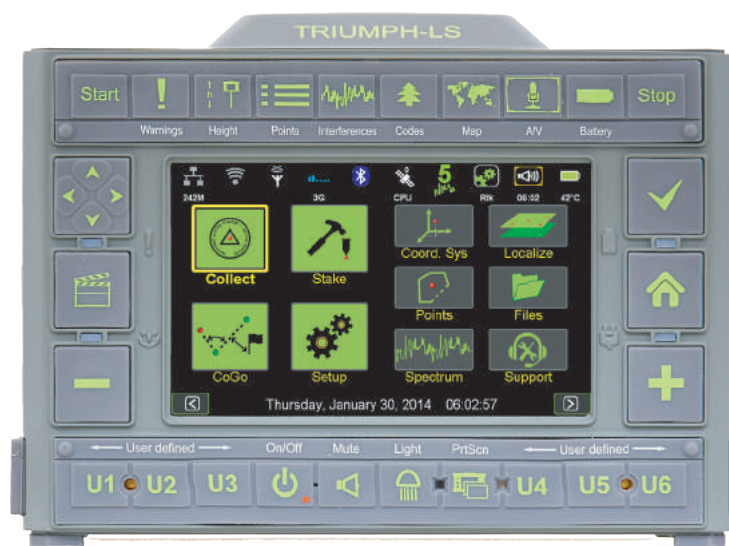
Рисунок 1. ТРИУМФ-ЛС
