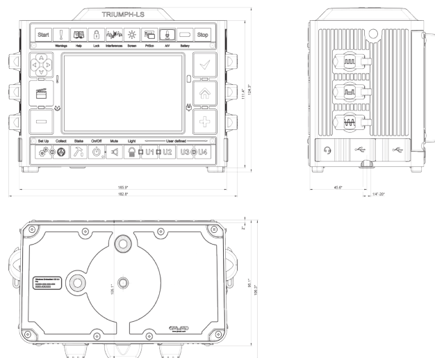
Рисунок 2. Габариты в мм
