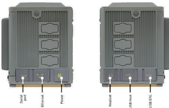
Рисунок 3. Порты приемника
